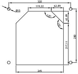
UNI-MAX OTWARTY 100kW
