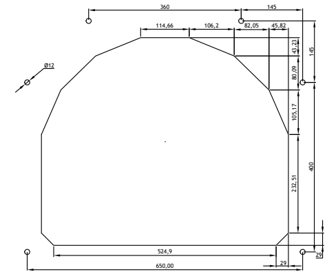
UNI-MAX OTWARTY 750kW
