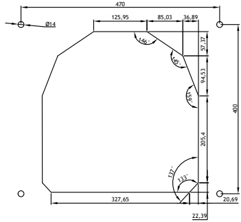
UNI-MAX OTWARTY 300kW
