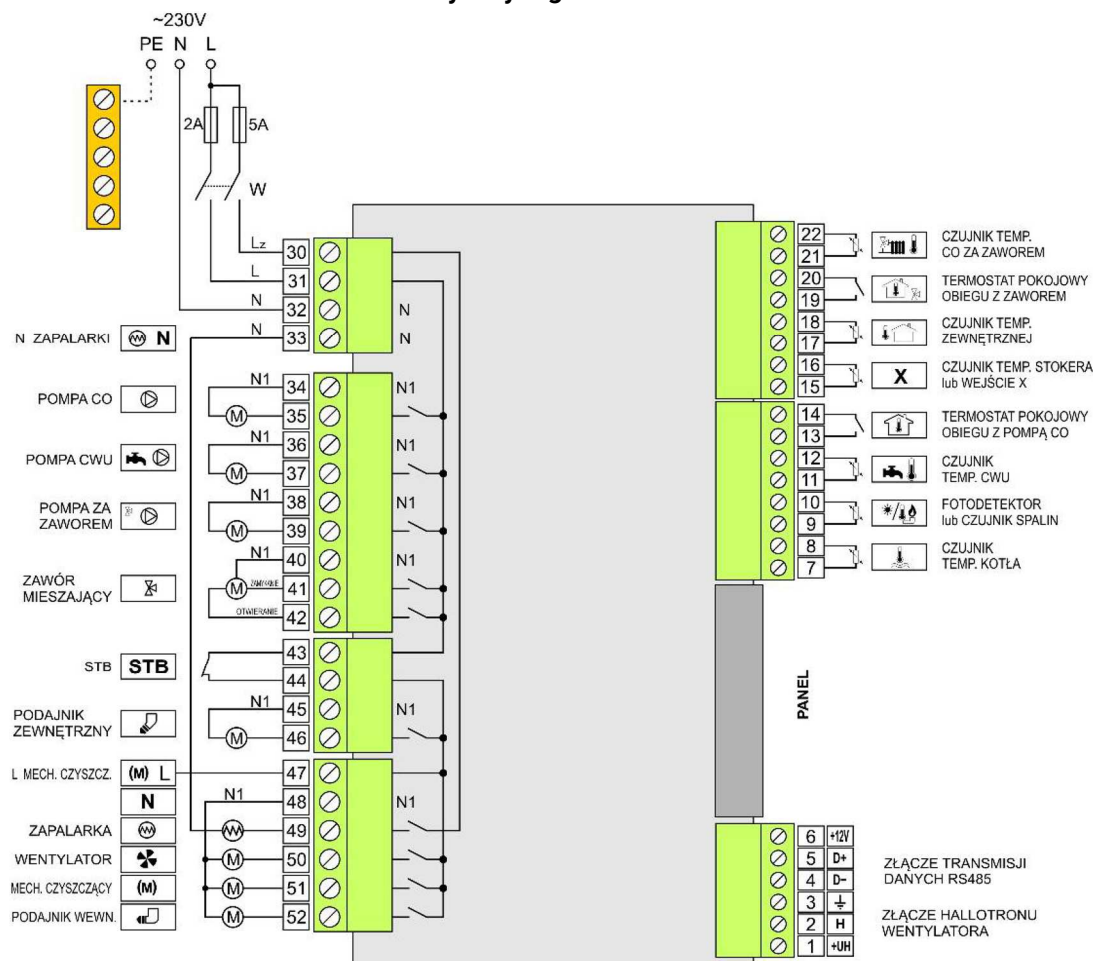
SCHEMAT WEJŚĆ ORAZ WYJŚĆ STEROWNIKA RK-2008SPGM
