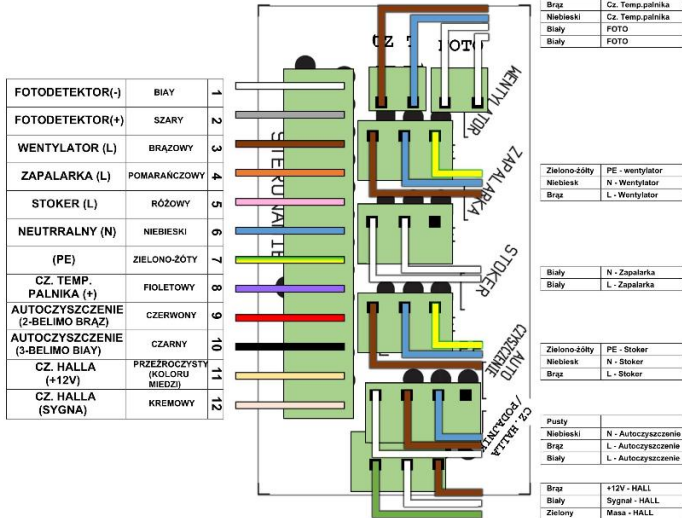
Schemat podłączenia regulatora RK-2008LPG/LPG2 do złącza palnika 12 pin
