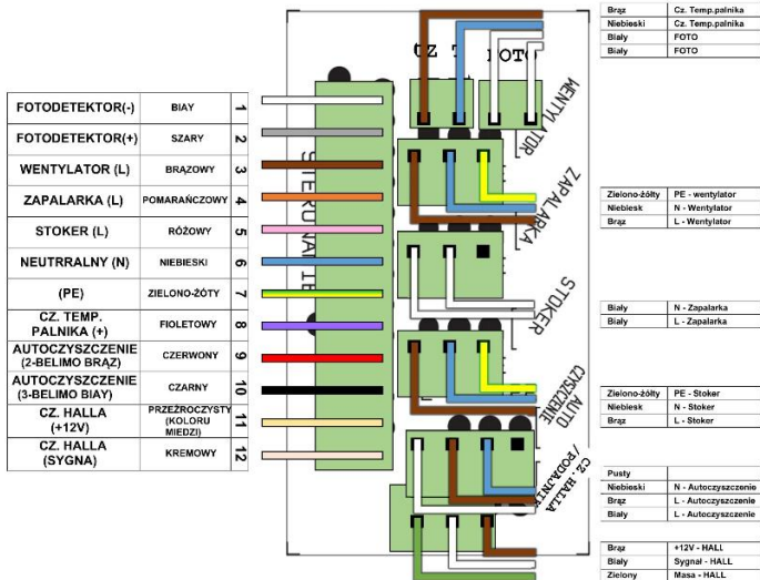
Schemat podłączenia regulatora RK-2008LPG/LPG2 do złącza palnika 12 pin
