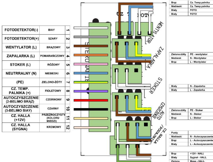
Schemat podłączenia regulatora RK-2008LPGW/LPG2W do złącza palnika 12 pin
